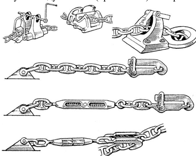
Рис. 9-7. Палубные стопоры.
