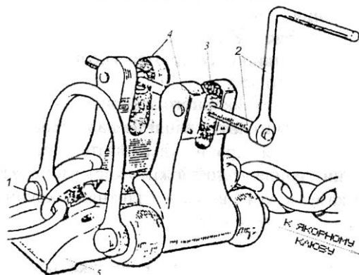
Рис. 9-7. Палубные стопоры.
